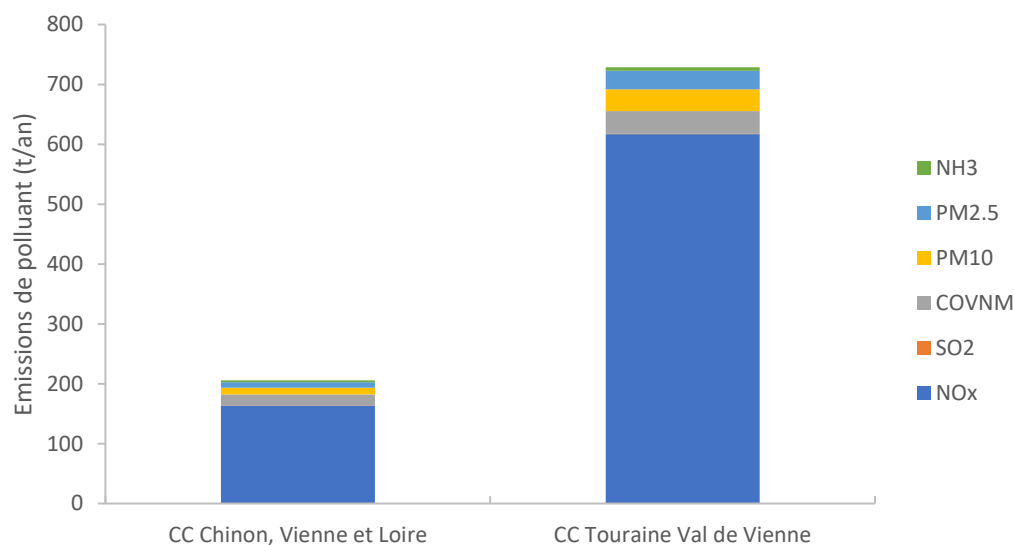
Figure 43 : Emissions de polluants atmosphériques liées au secteur du transport routier
