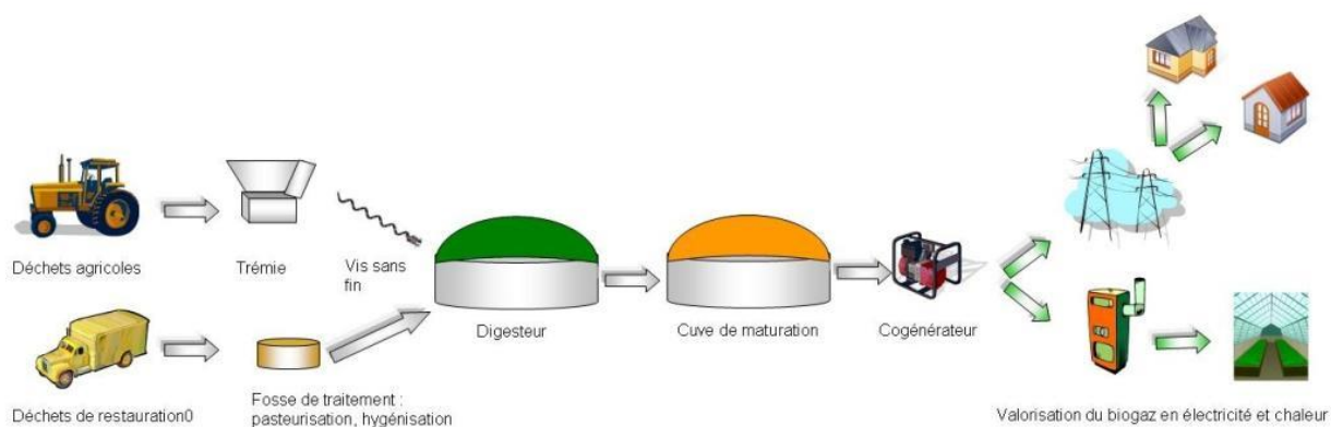
Figure 77 : Descriptif du procédé de méthanisation
