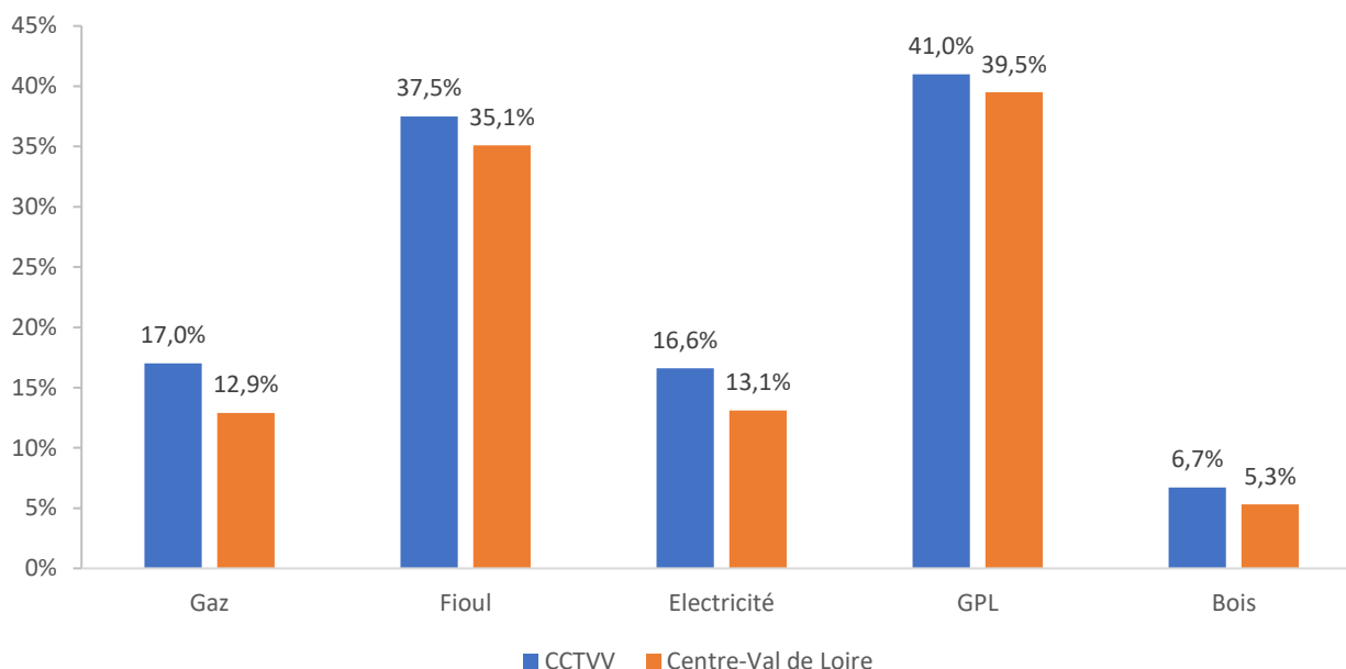
Figure 60 : Part des ménages ayant un TEE Logement > 10% des revenus disponibles selon l'énergie de chauffage (%) – Source : PRECARITER, Energies Demain, propriété d'Enedis – 2012
