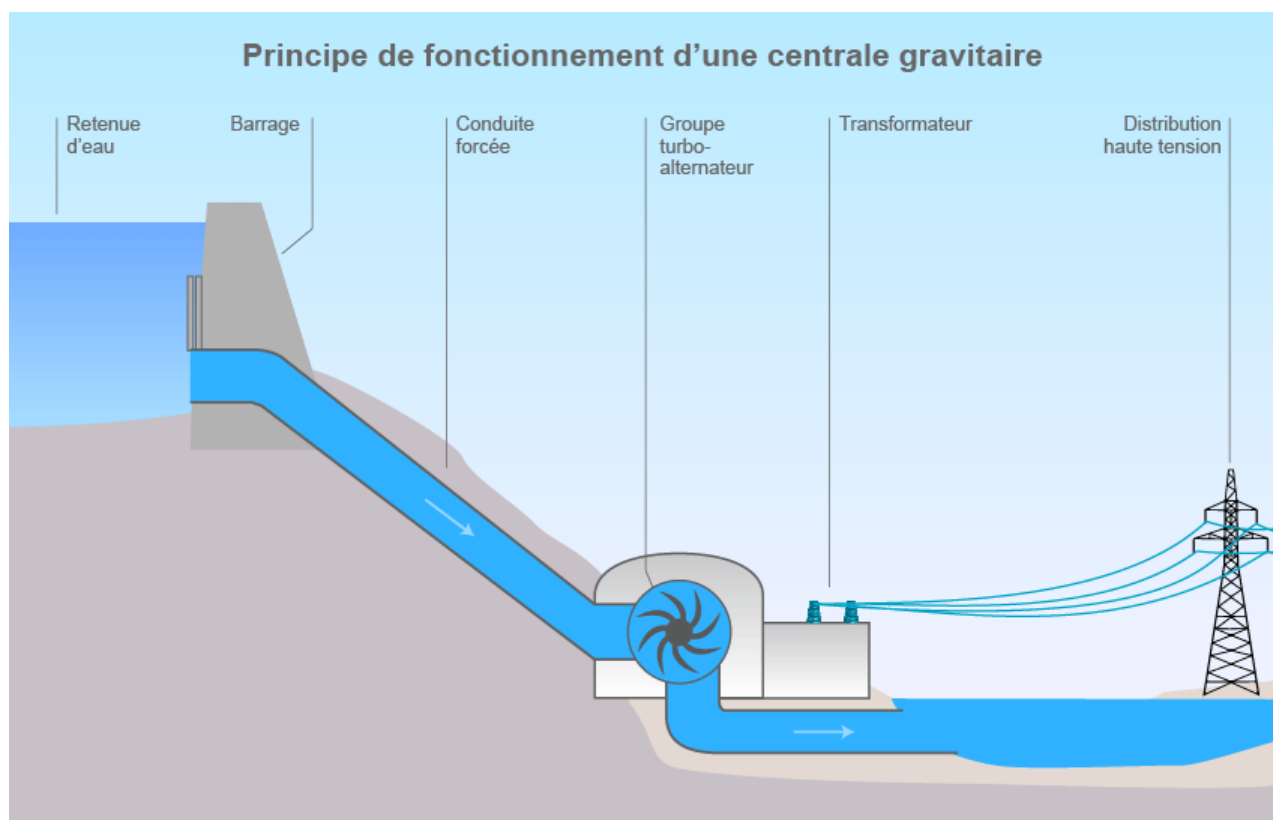
Figure 95 : Schéma de principe d'une centrale gravitaire
