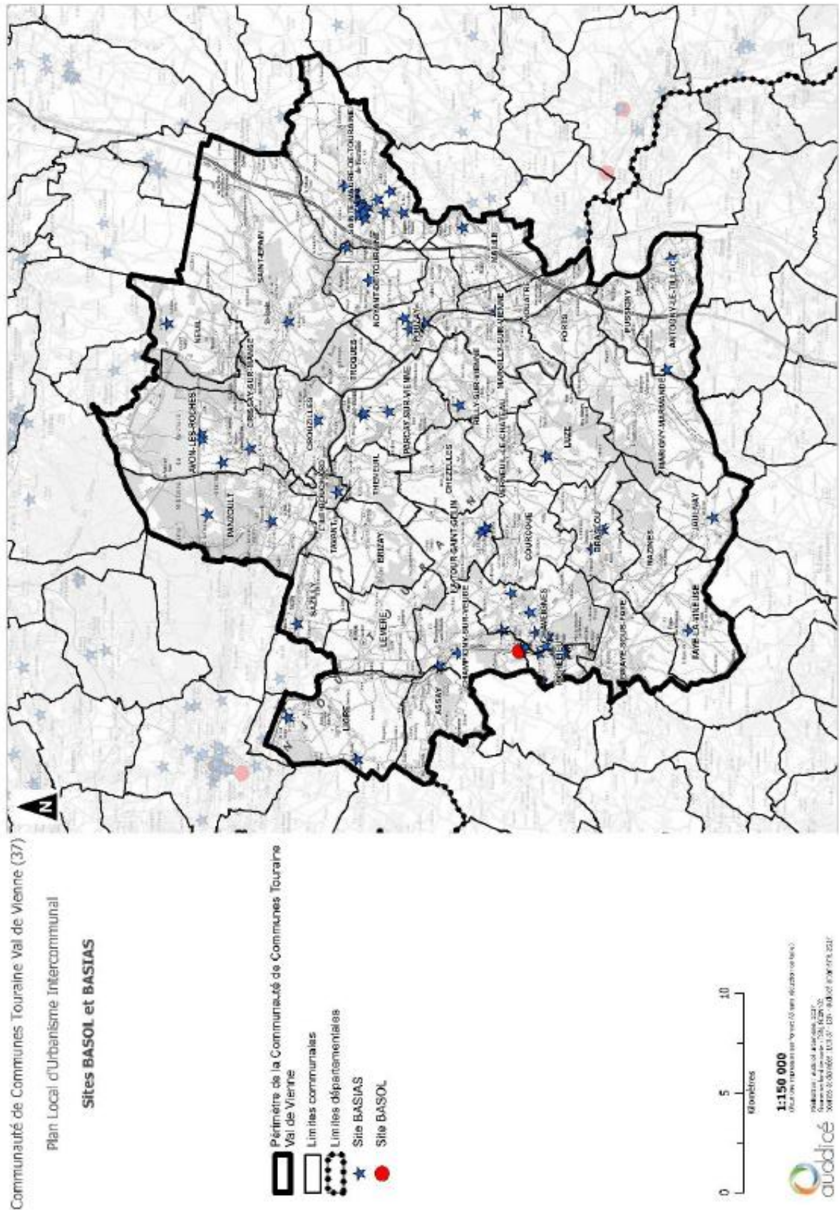
Carte 80 : Les sites BASIAS et BASOL de la CCTVV – source : DDT 37
