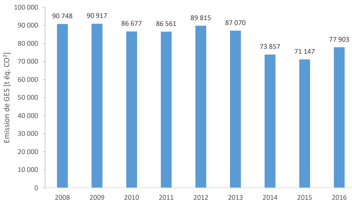
Figure 20 : Emissions de gaz à effet de serre de CCCVL - Source : LIG'Air
