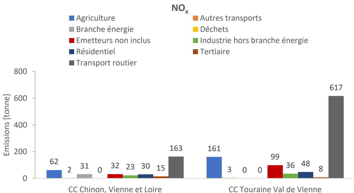
Figure 29 : Répartition sectorielle des émissions d'oxydes d'azote (NO x ) en 2012 - Source : LIG'AIR
