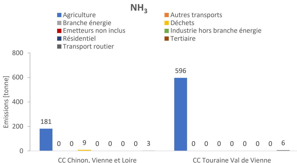
Figure 35 : Répartition sectorielle des émissions d'ammoniac en 2012 - Source : LIG'AIR
