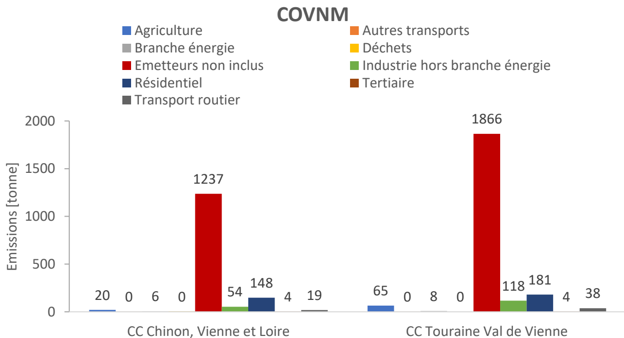
Figure 31 : Répartition sectorielle des émissions de COVNM en 2012 - Source : LIG'AIR
