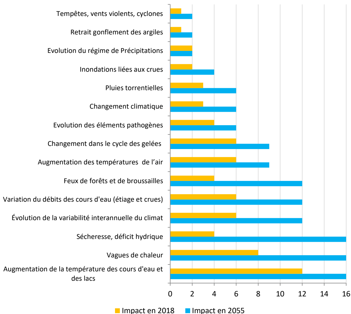
Figure 118 : Classement des aléas climatiques par note de vulnérabilité pour les territoires du PNR LAT (Source : PNR LAT)
