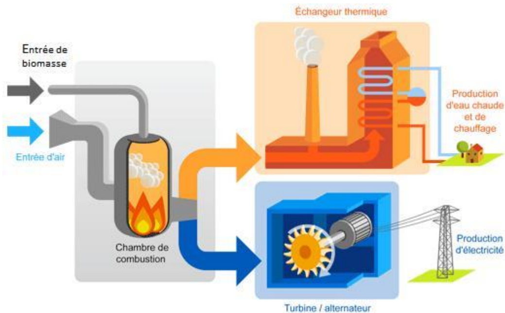
Figure 89 : Schéma de principe de la cogénération - Source : EDF
