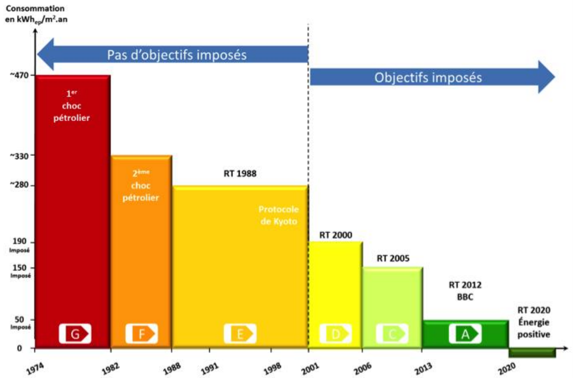
Figure 45 : Historique des réglementations thermiques – Source : CFBP
