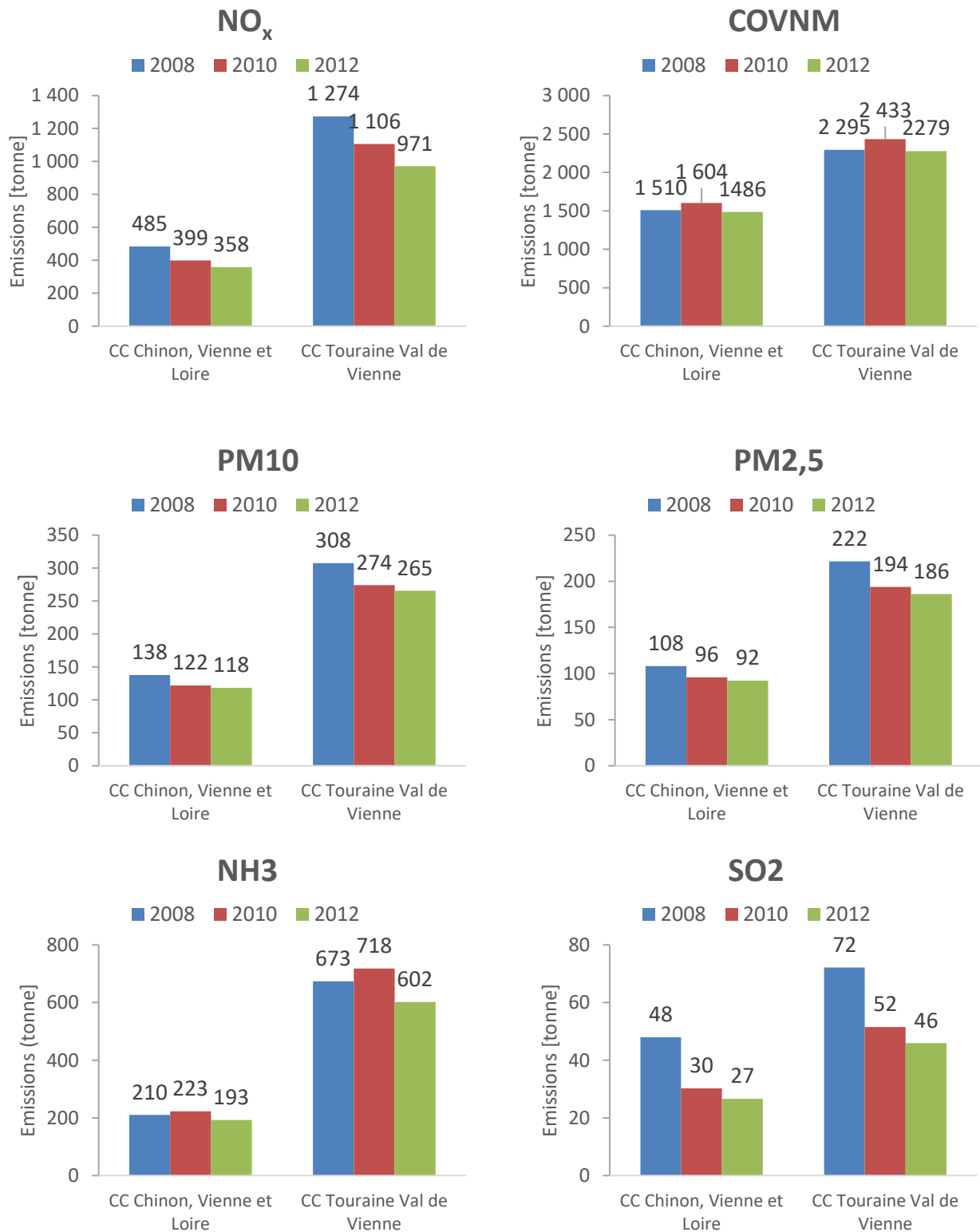
Figure 28 : Evolution des émissions de polluants atmosphériques de 2008 à 2012 - Source : LIG'AIR
