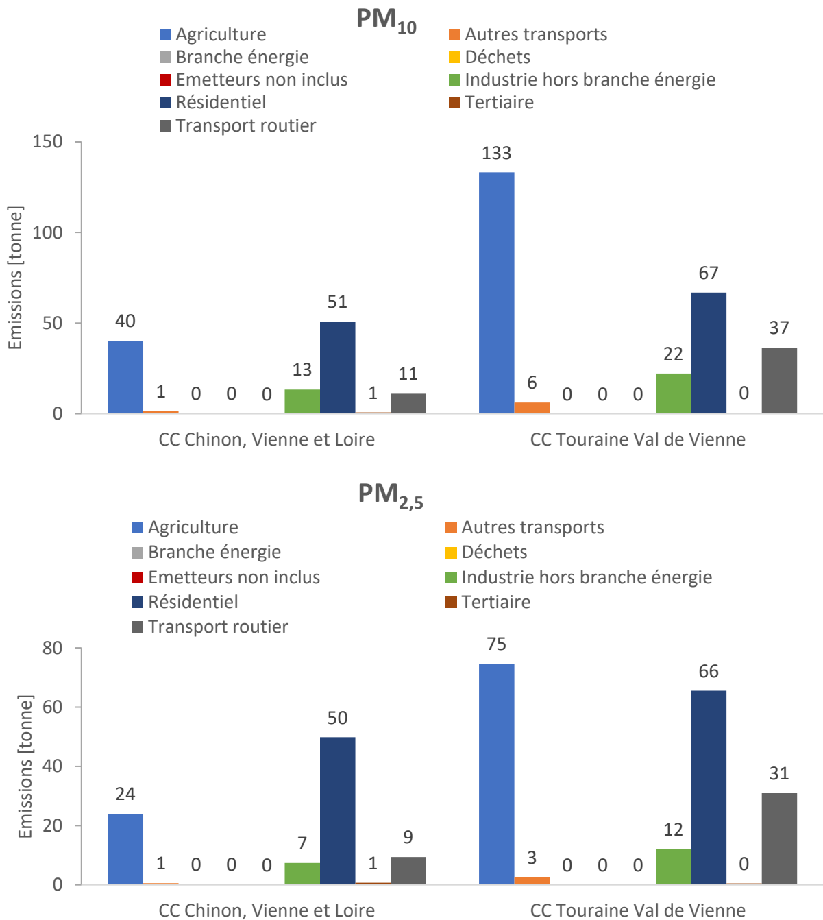
Figure 32 : Répartition sectorielle des émissions de particules fines en 2012 - Source : LIG'Air
