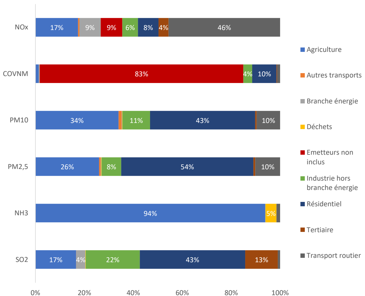
Figure 37 : Répartition des contributions des différents secteurs aux émissions de polluants atmosphériques sur la CC CVL - Source : LIG'AIR
