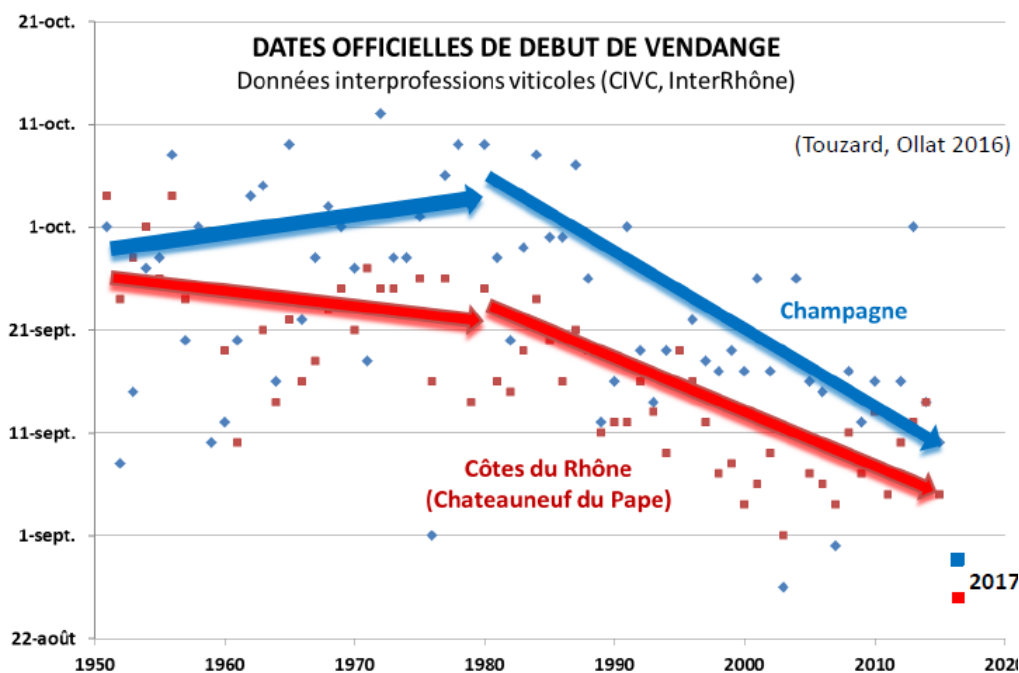
Figure 120 : Dates officielles des dates de début de vendange entre 1950 et 2017 (Source : Touzard, Ollat 2016 dans Vendramini Busnot-Richard 2017)
