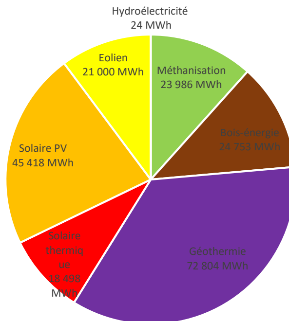
Figure 96 : Répartition des potentiels supplémentaires mobilisables en énergies renouvelables sur la CCCVL
